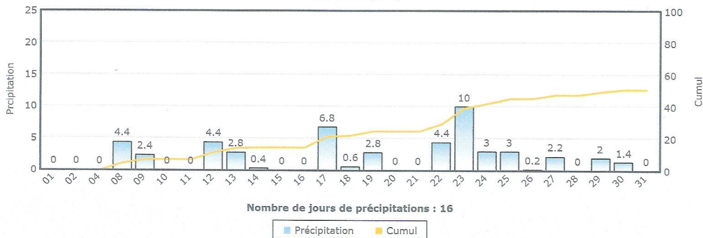
Précipitation (mm)
