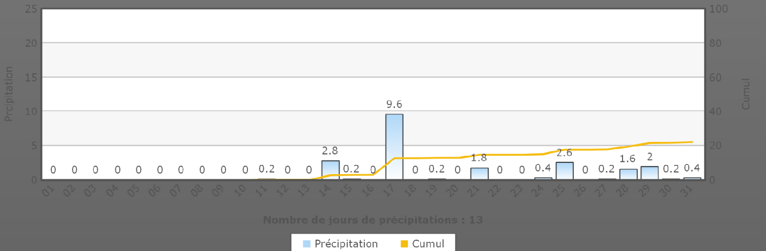
Précipitation (mm)
